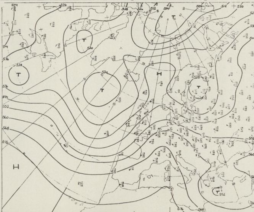
Höhenwetterkarte (Absolute Topographie 500 mb entsprechend ca. 5500 m Höhe) vom 09.02. 01 Uhr
