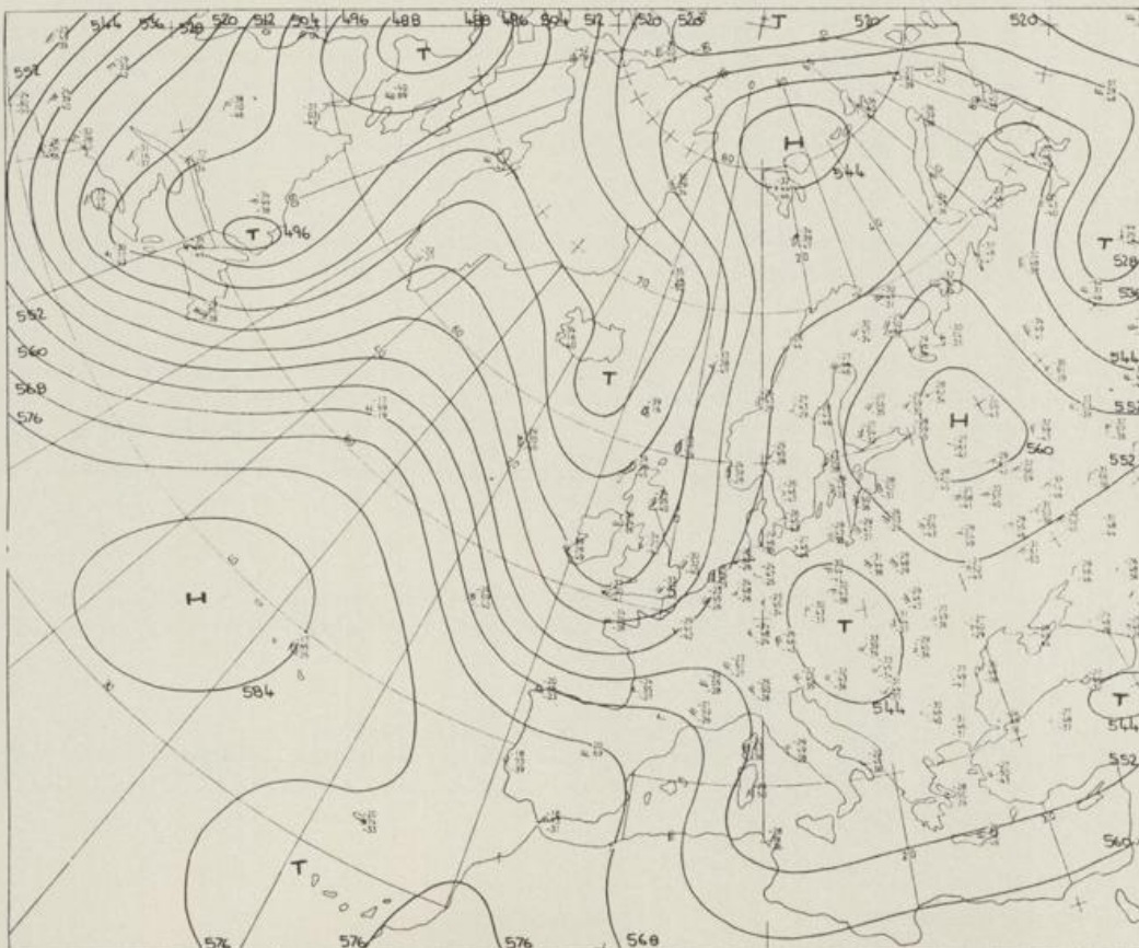
Höhenwetterkarte (Absolute Topographie 500 mb entsprechend ca. 5500 m Höhe) vom 13.03. 01 Uhr
