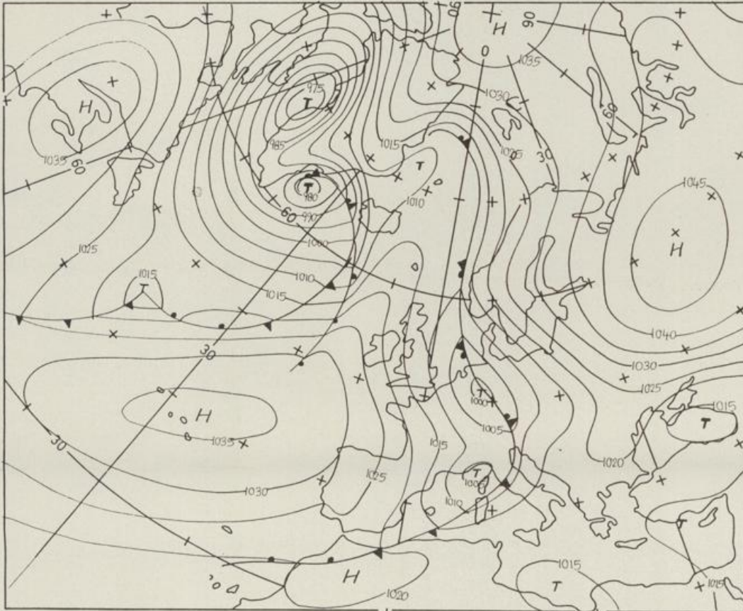
Bodenwetterkarte Vorhersage für den 14.03. 01 Uhr
