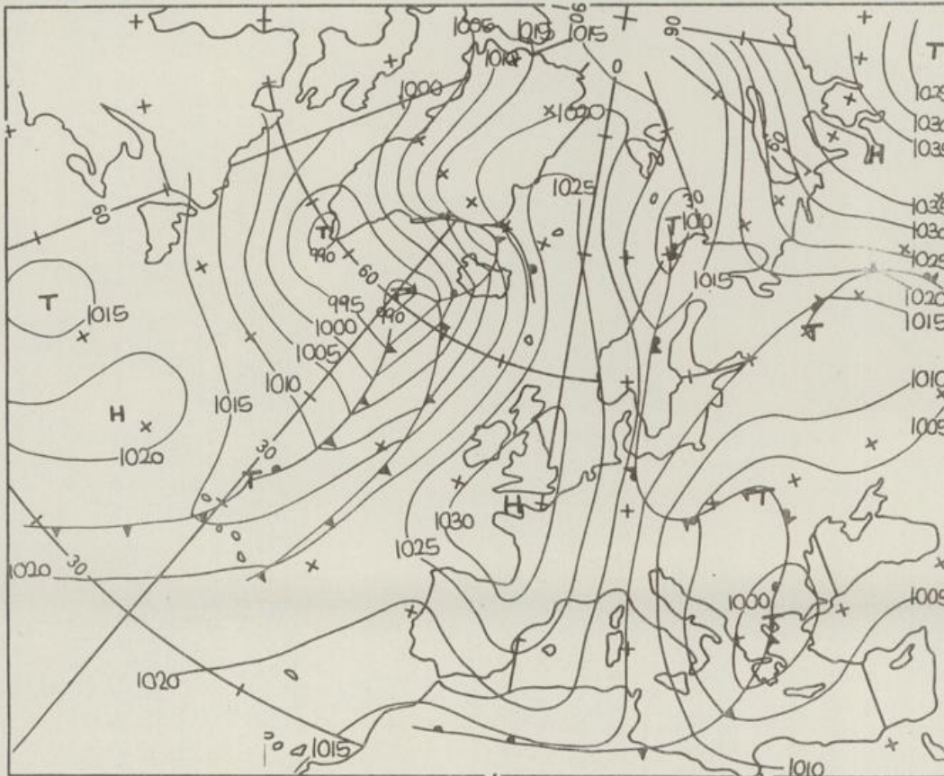
Bodenwetterkarte Vorhersage für den 04.03. 01 Uhr
