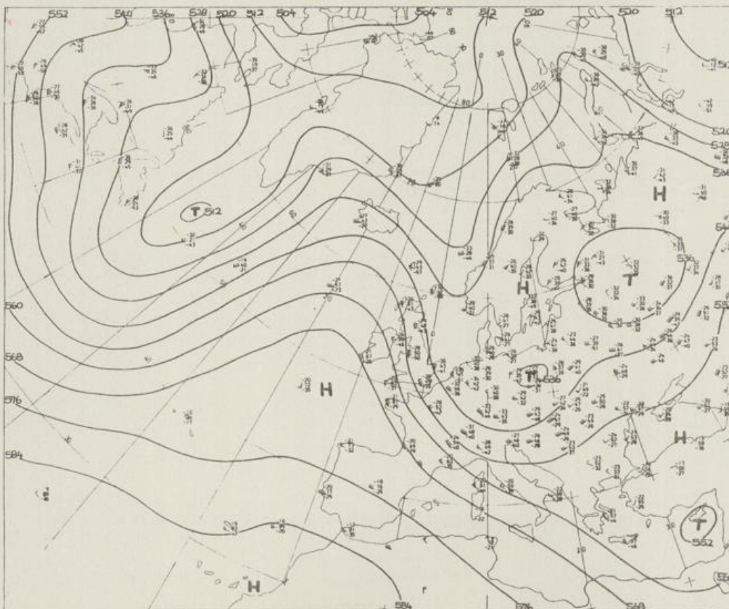
Höhenwetterkarte (Absolute Topographie 500 mb entsprechend ca. 5500 m Höhe) vom 03.03. 01 Uhr
