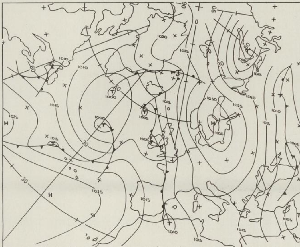
Bodenwetterkarte Vorhersage für den 13.05. 02 Uhr
