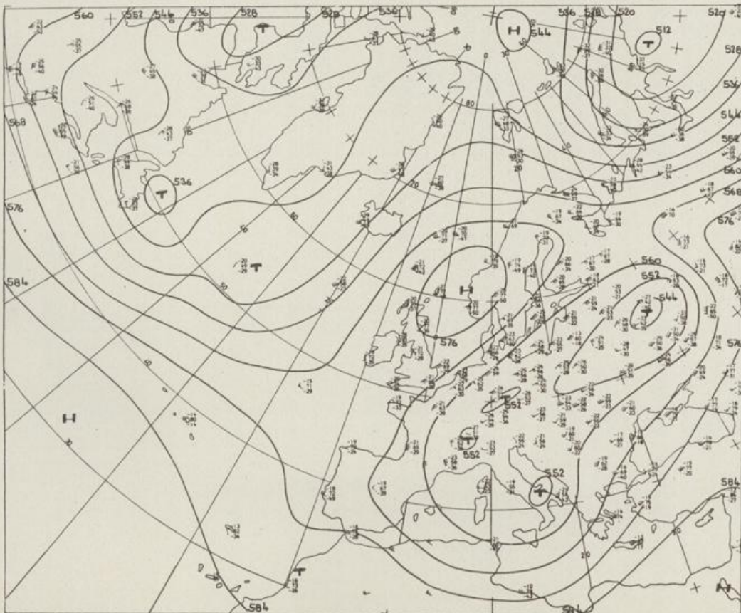
Höhenwetterkarte (Absolute Topographie 500 mb entsprechend ca. 5500 m Höhe) vom 16.05. 02 Uhr
