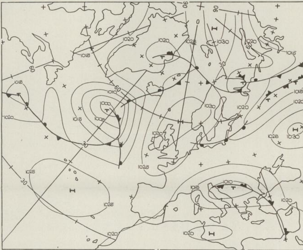
Bodenwetterkarte Vorhersage für den 17.05. 02 Uhr
