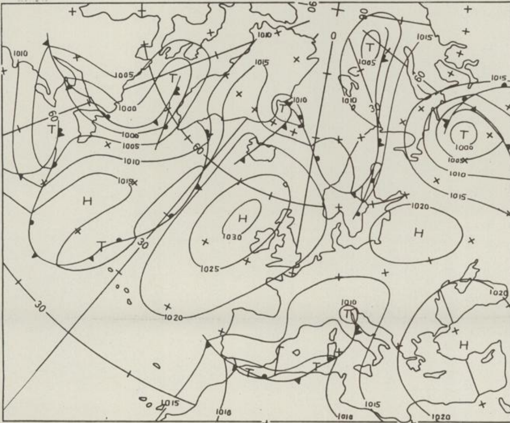
Bodenwetterkarte Vorhersage für den 23.05. 02 Uhr
