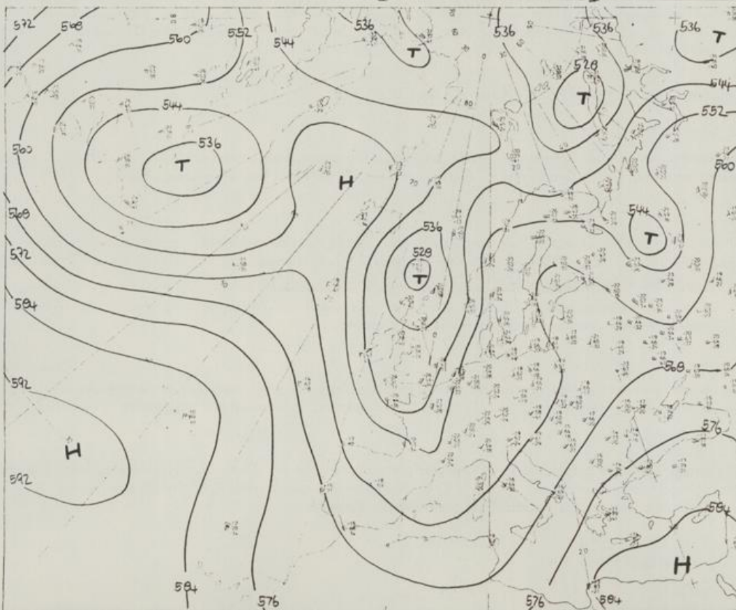
Höhenwetterkarte (Absolute Topographie 500 mb entsprechend ca. 5500 m Höhe) vom 29.05. 02 Uhr
