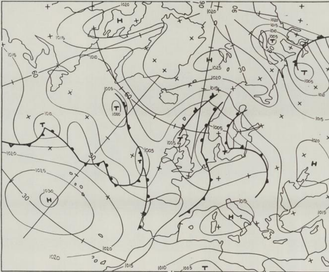
Bodenwetterkarte Vorhersage für den 30.05. 02 Uhr
