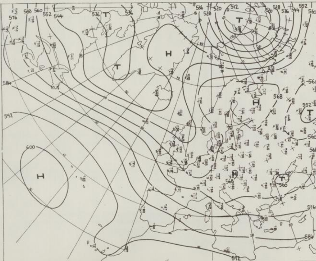
Höhenwetterkarte (Absolute Topographie 500 mb entsprechend ca. 5500 m Höhe) vom 18.06. 02 Uhr
