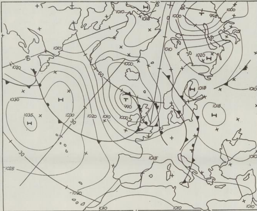
Bodenwetterkarte Vorhersage für den 19.06. 02 Uhr
