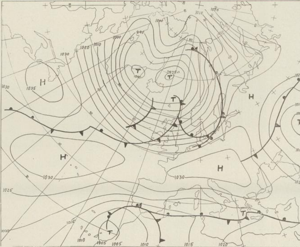
Bodenwetterkarte Vorhersage für den 07.01. 01 Uhr
