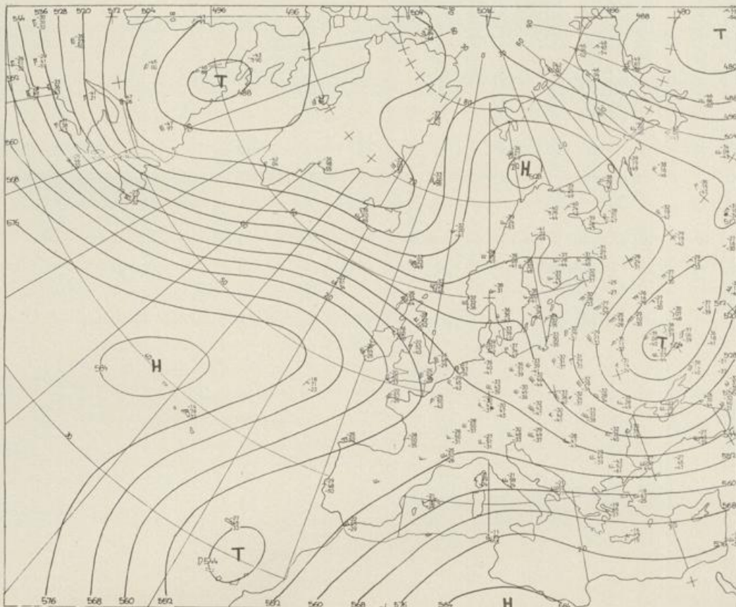
Höhenwetterkarte (Absolute Topographie 500 mb entsprechend ca. 5500 m Höhe) vom 06.01. 01 Uhr
