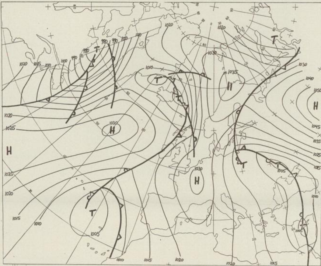
Bodenwetterkarte Vorhersage für den 16.01. 01 Uhr
