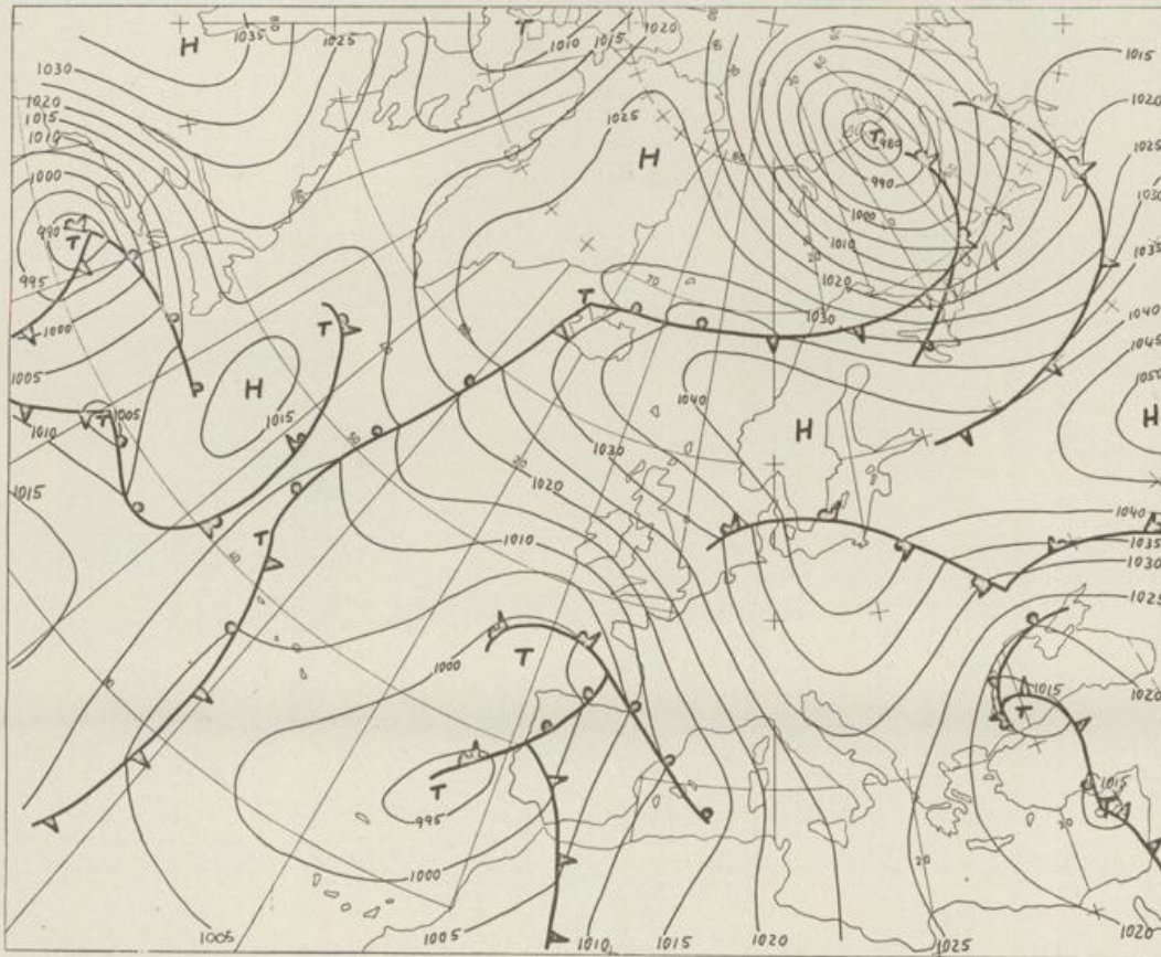
Bodenwetterkarte Vorhersage für den 19.01. 01 Uhr
