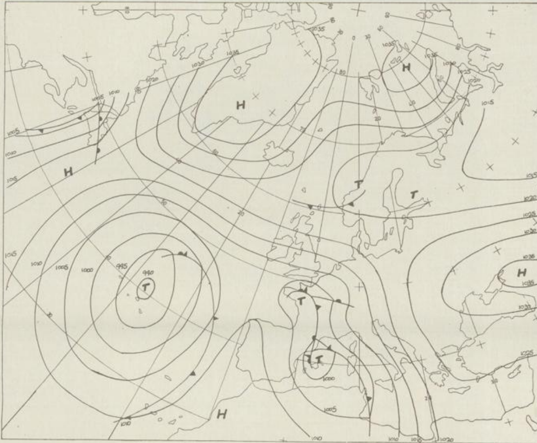
Bodenwetterkarte Vorhersage für den 23.01. 01 Uhr
