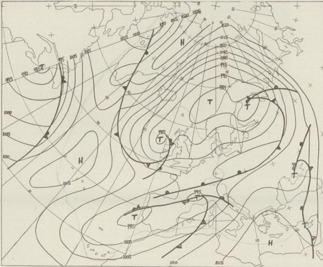
Bodenwetterkarte Vorhersage für den 28.01. 01 Uhr
