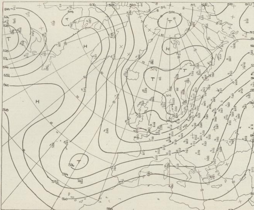
Höhenwetterkarte (Absolute Topographie 500 mb entsprechend ca. 5500 m Höhe) vom 27.01. 01 Uhr
