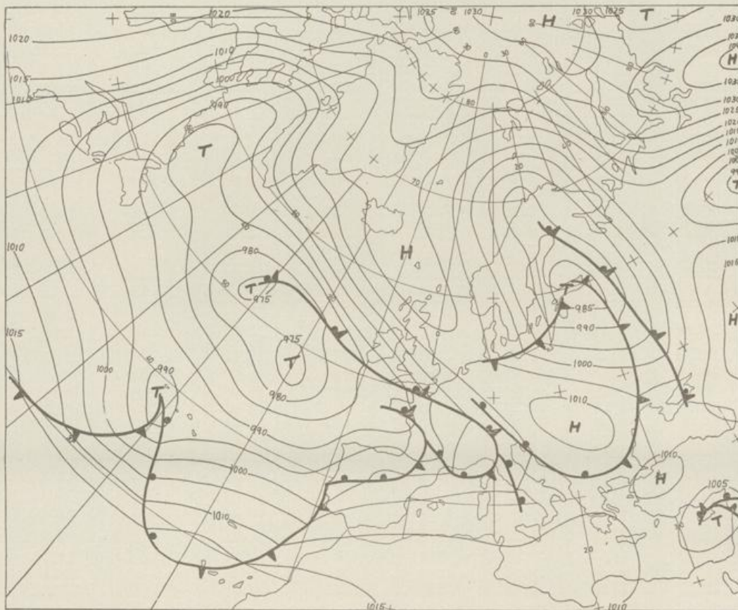
Bodenwetterkarte Vorhersage für den 10.02. 01 Uhr
