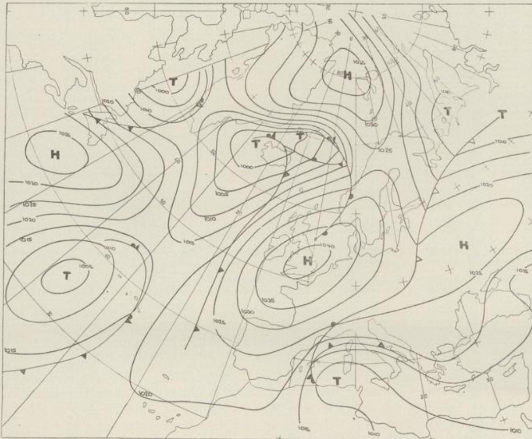
Bodenwetterkarte Vorhersage für den 25.02. 01 Uhr
