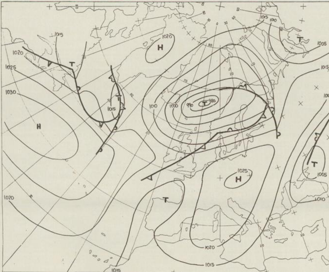
Bodenwetterkarte Vorhersage für den 15.05. 01 Uhr
