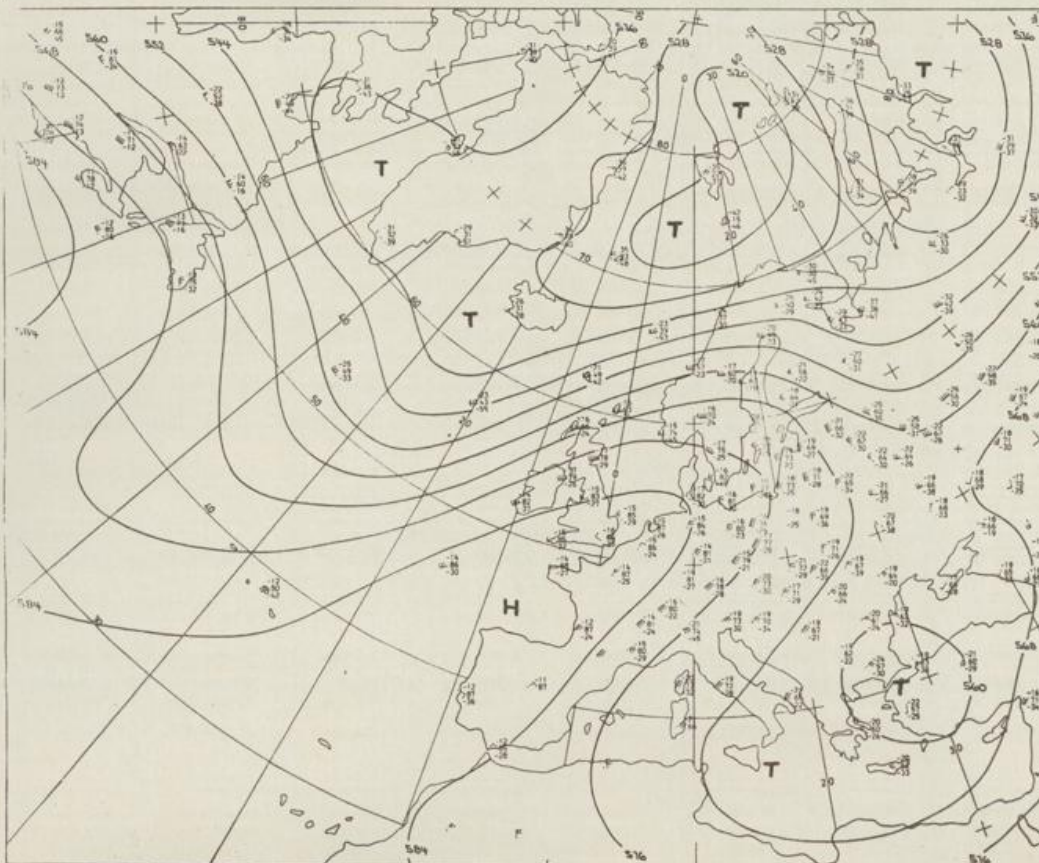
Höhenwetterkarte (Absolute Topographie 500 mb entsprechend ca. 5500 m Höhe) vom 14.05. 01 Uhr
