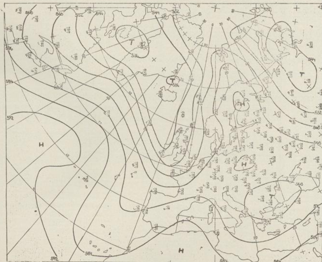
Höhenwetterkarte (Absolute Topographie 500 mb entsprechend ca. 5500 m Höhe) vom 24.06. 01 Uhr
