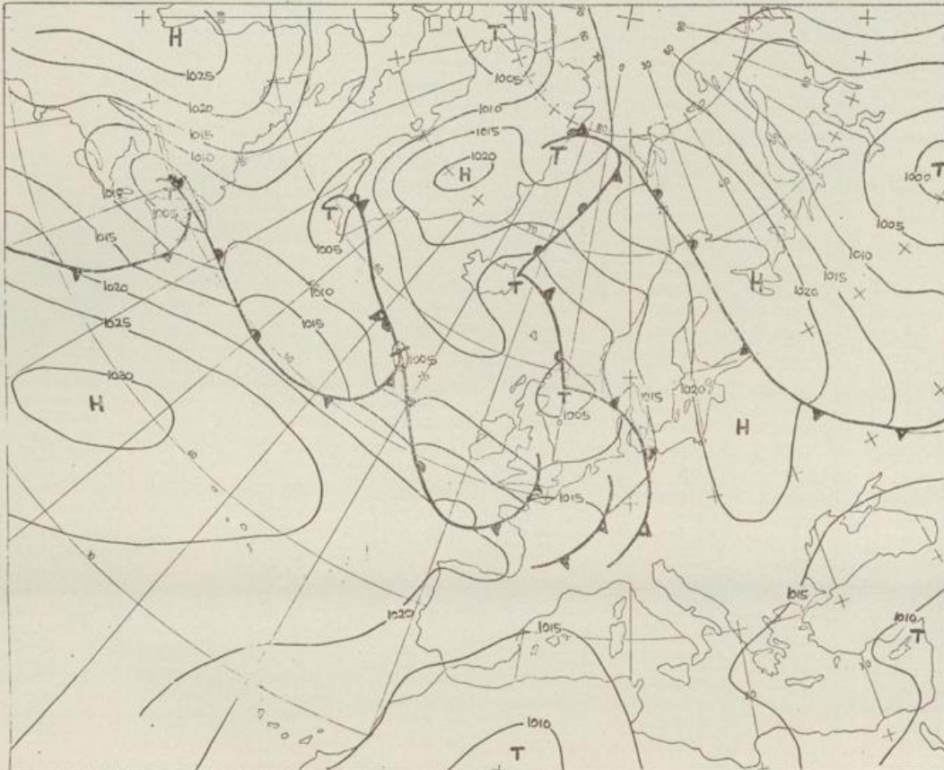
Bodenwetterkarte Vorhersage für den 25.06. 01 Uhr
