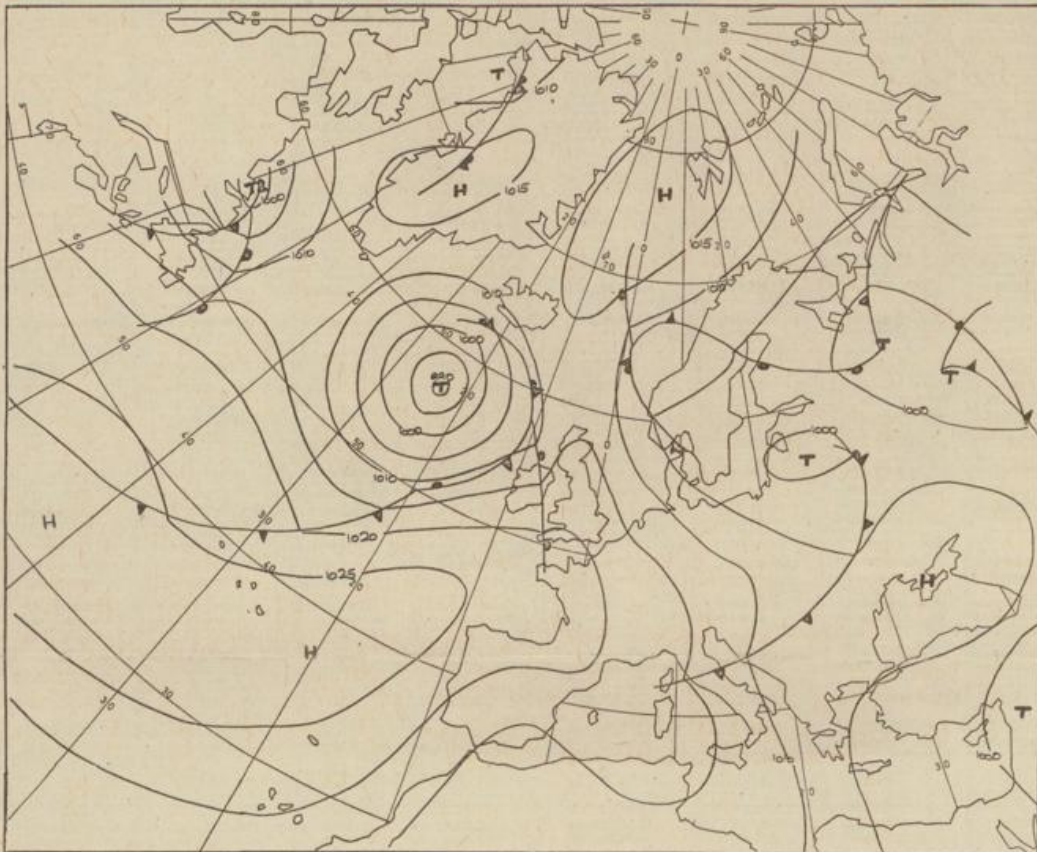
Bodenwetterkarte Vorhersage für den 22.07. 01 Uhr
