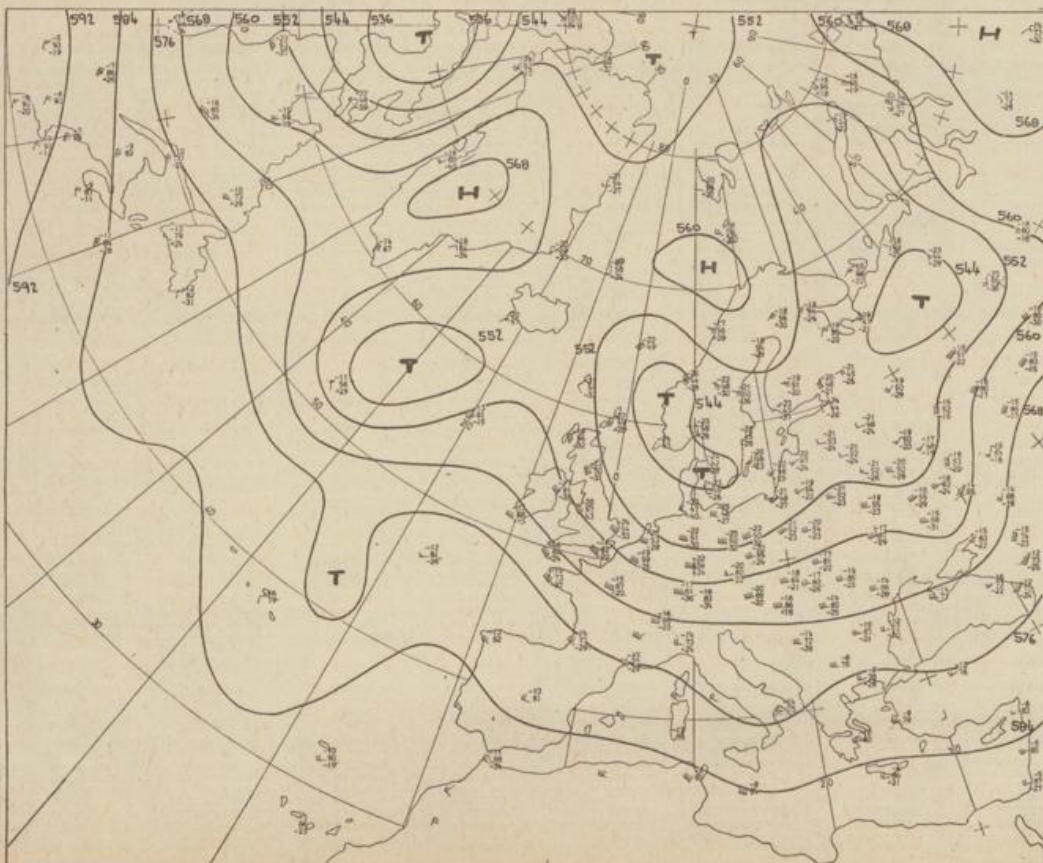
Höhenwetterkarte (Absolute Topographie 500 mb entsprechend ca. 5500 m Höhe) vom 21.07. 01 Uhr
