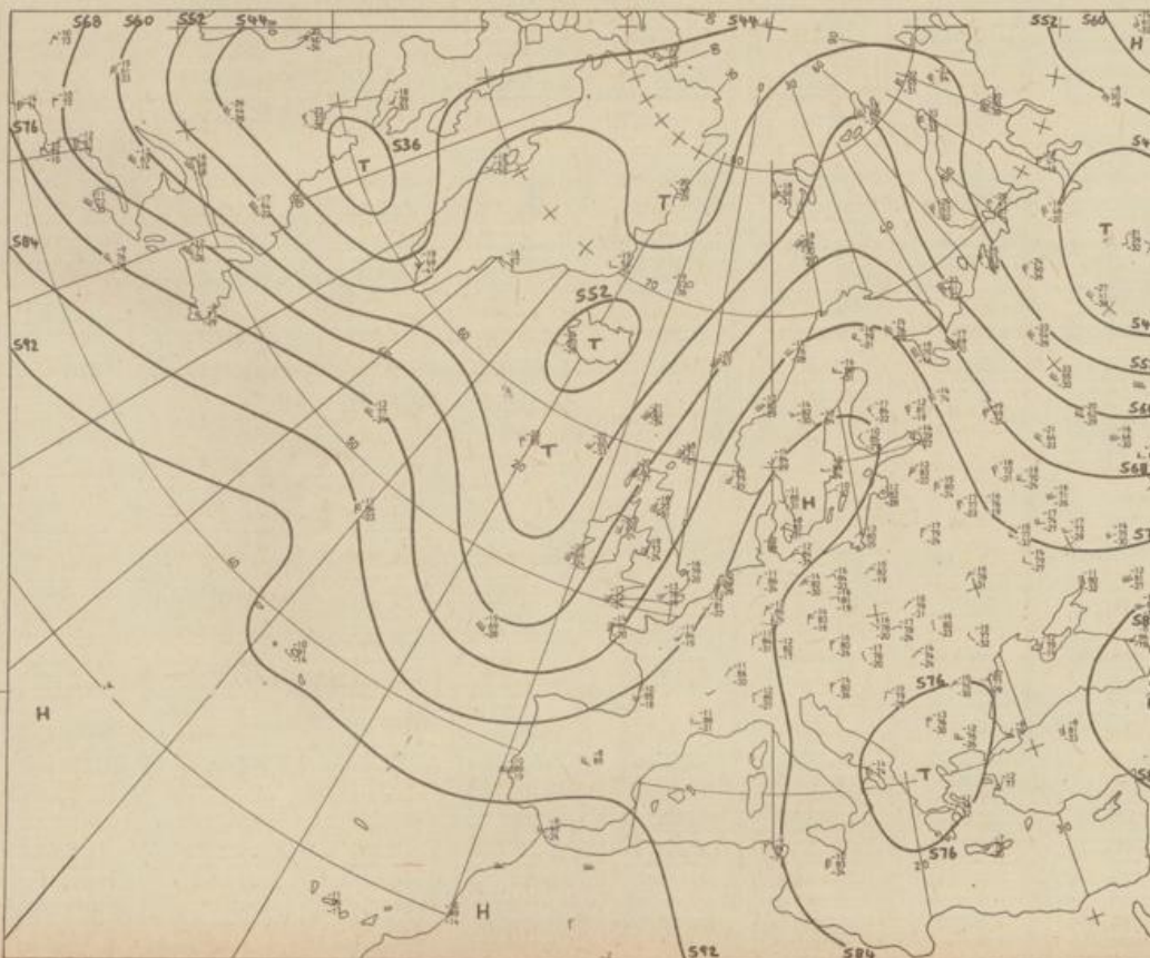
Höhenwetterkarte (Absolute Topographie 500 mb entsprechend ca. 5500 m Höhe) vom 30.07. 01 Uhr
