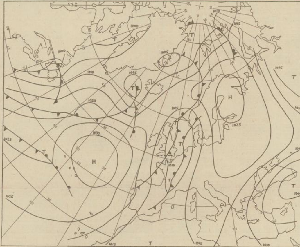
Bodenwetterkarte Vorhersage für den 31.07. 01 Uhr
