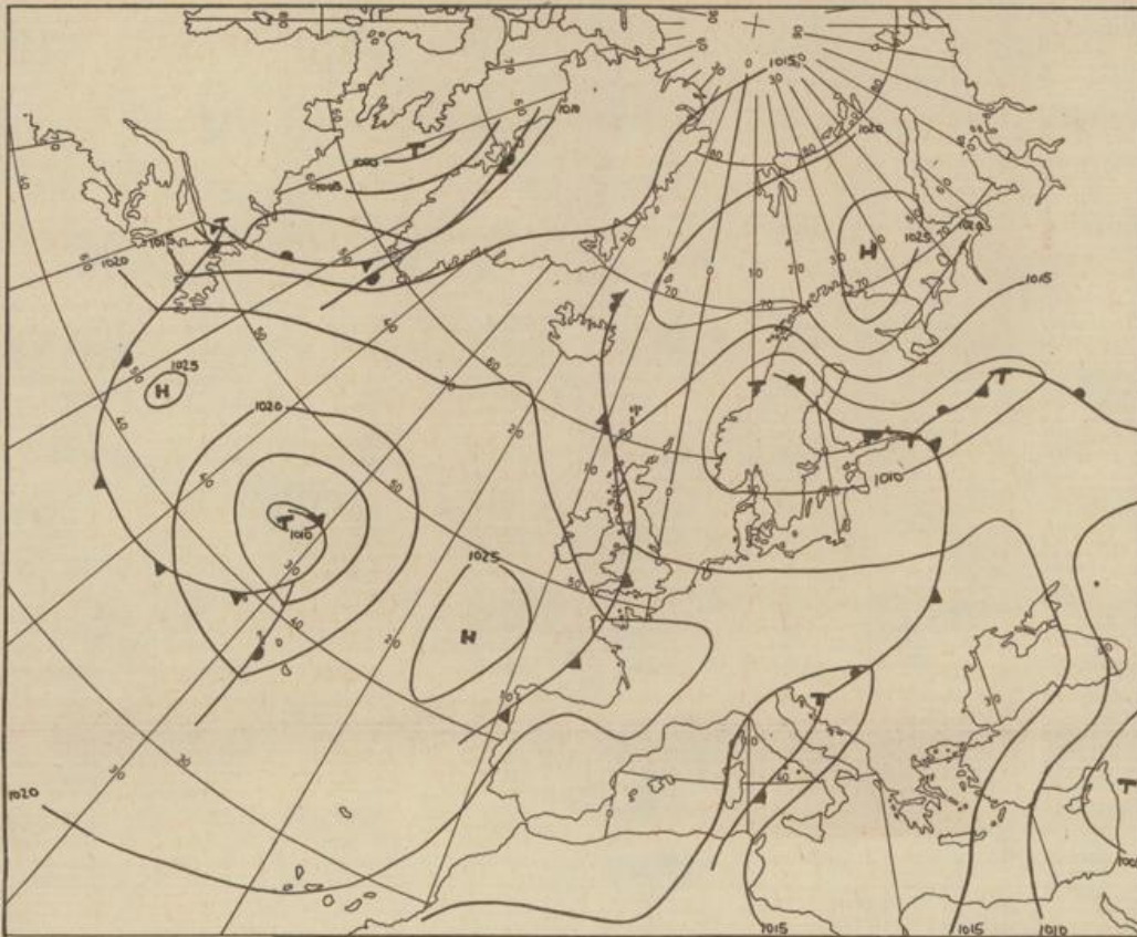
Bodenwetterkarte Vorhersage für den 05.08. 01 Uhr
