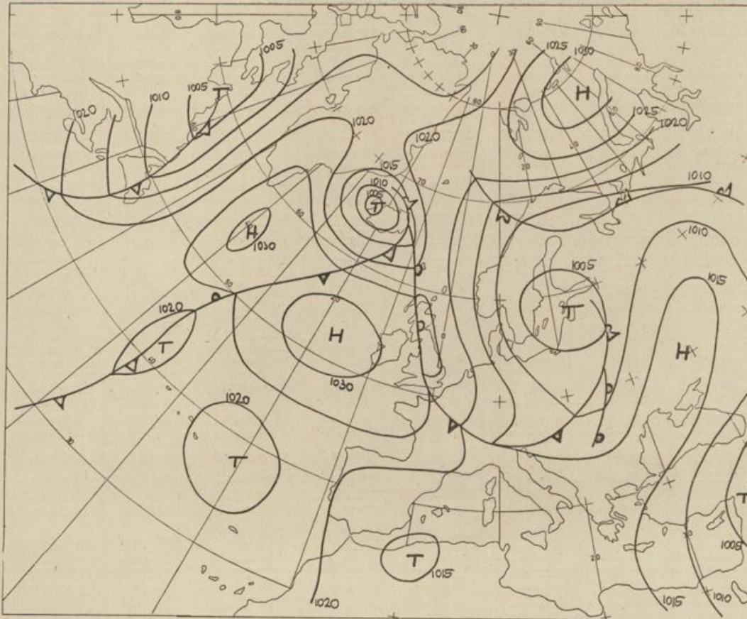
Bodenwetterkarte Vorhersage für den 31.08. 01 Uhr
