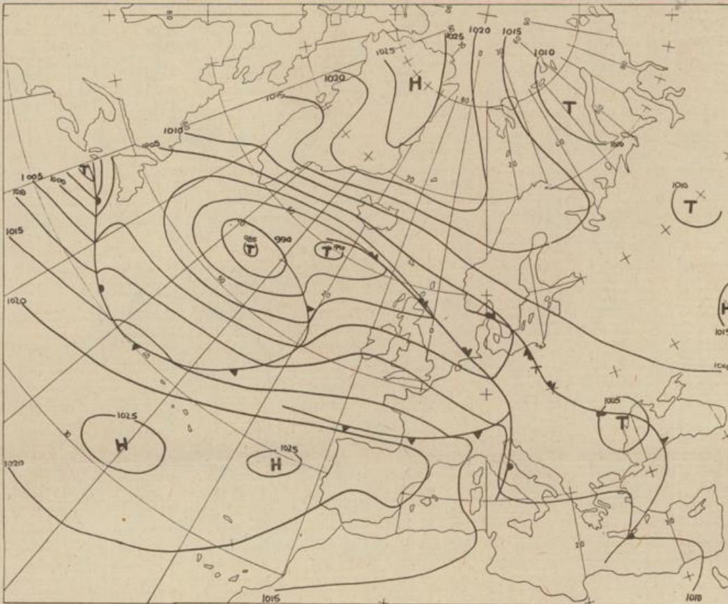
Bodenwetterkarte Vorhersage für den 08.09. 01 Uhr
