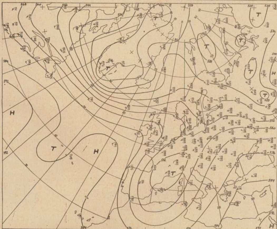
Höhenwetterkarte (Absolute Topographie 500 mb entsprechend ca. 5500 m Höhe) vom 02.10. 01 Uhr
