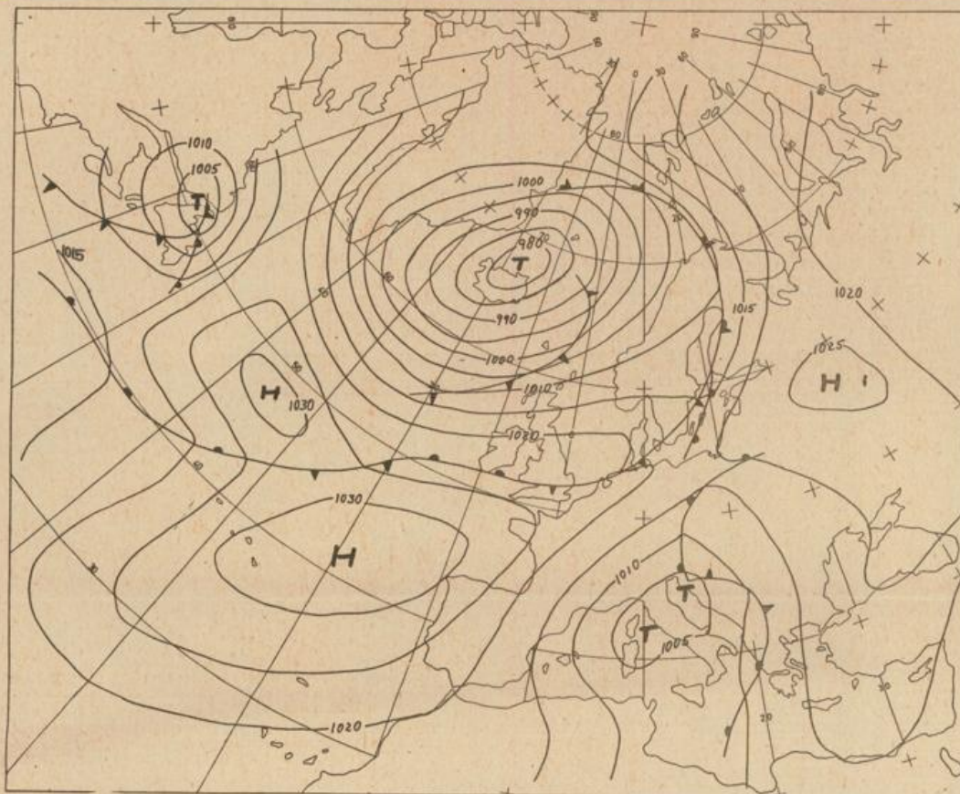
Bodenwetterkarte Vorhersage für den 03.10. 01 Uhr
