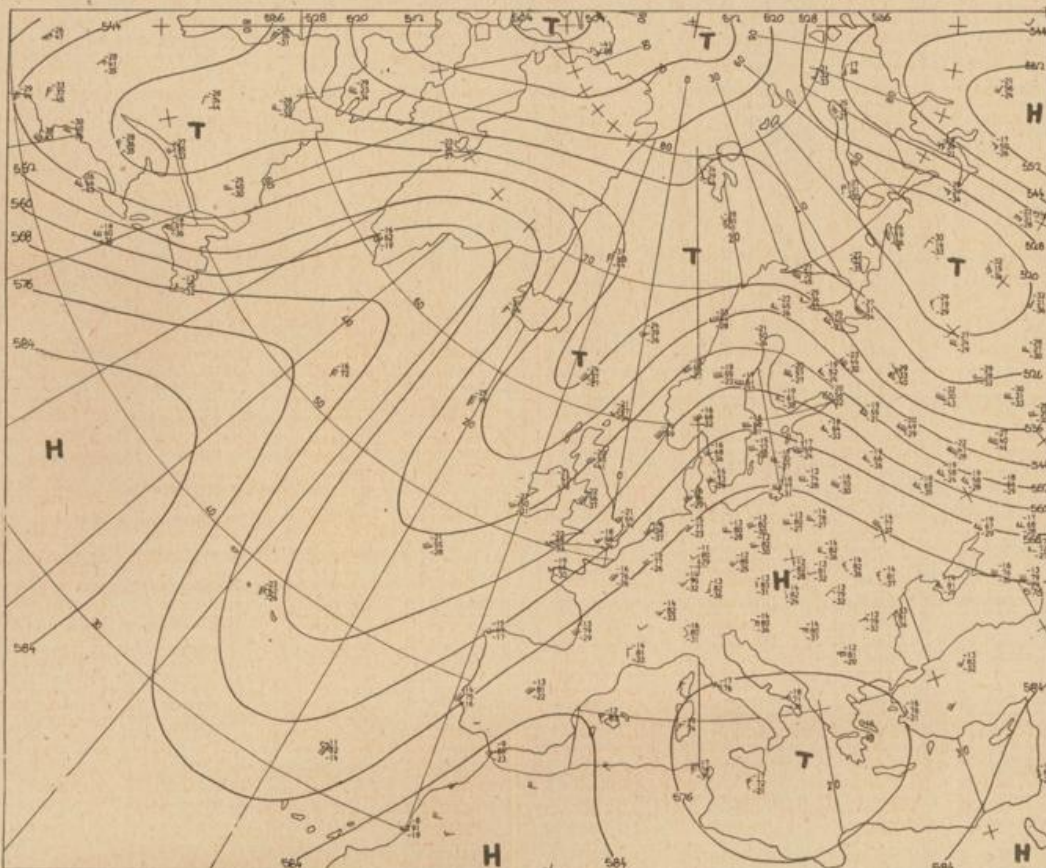
Höhenwetterkarte (Absolute Topographie 500 mb entsprechend ca. 5500 m Höhe) vom 09.10. 01 Uhr
