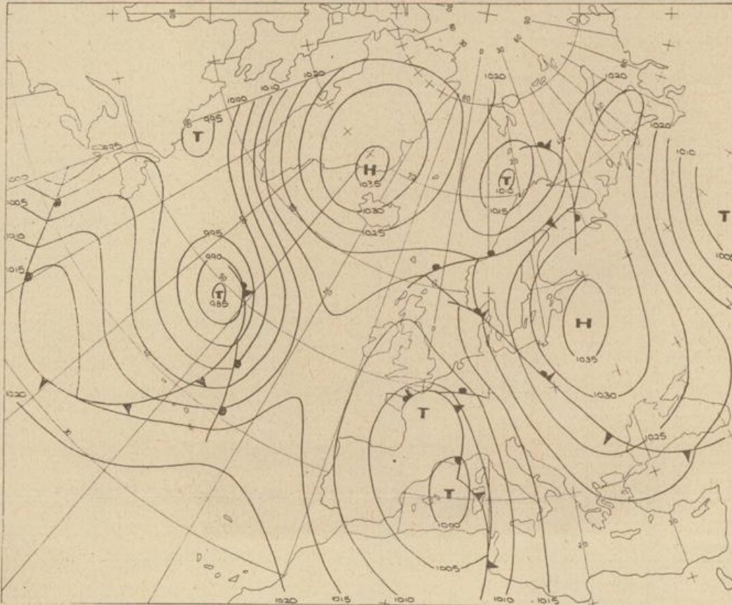
Bodenwetterkarte Vorhersage für den 22.12. 01 Uhr
