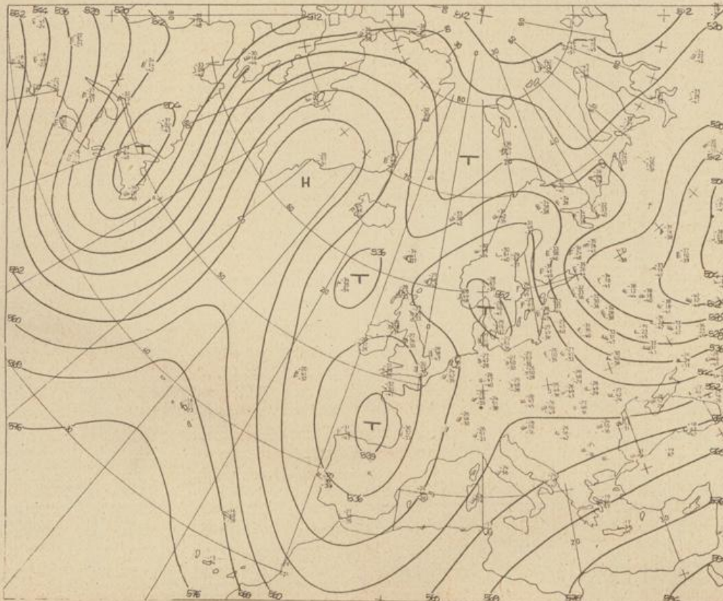
Höhenwetterkarte (Absolute Topographie 500 mb entsprechend ca. 5500 m Höhe) vom 21.12. 01 Uhr
