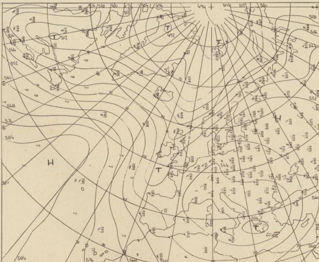
Höhenwetterkarte (Absolute Topographie 500 mb entsprechend ca. 5500 m Höhe) vom 12.4. 01 Uhr
