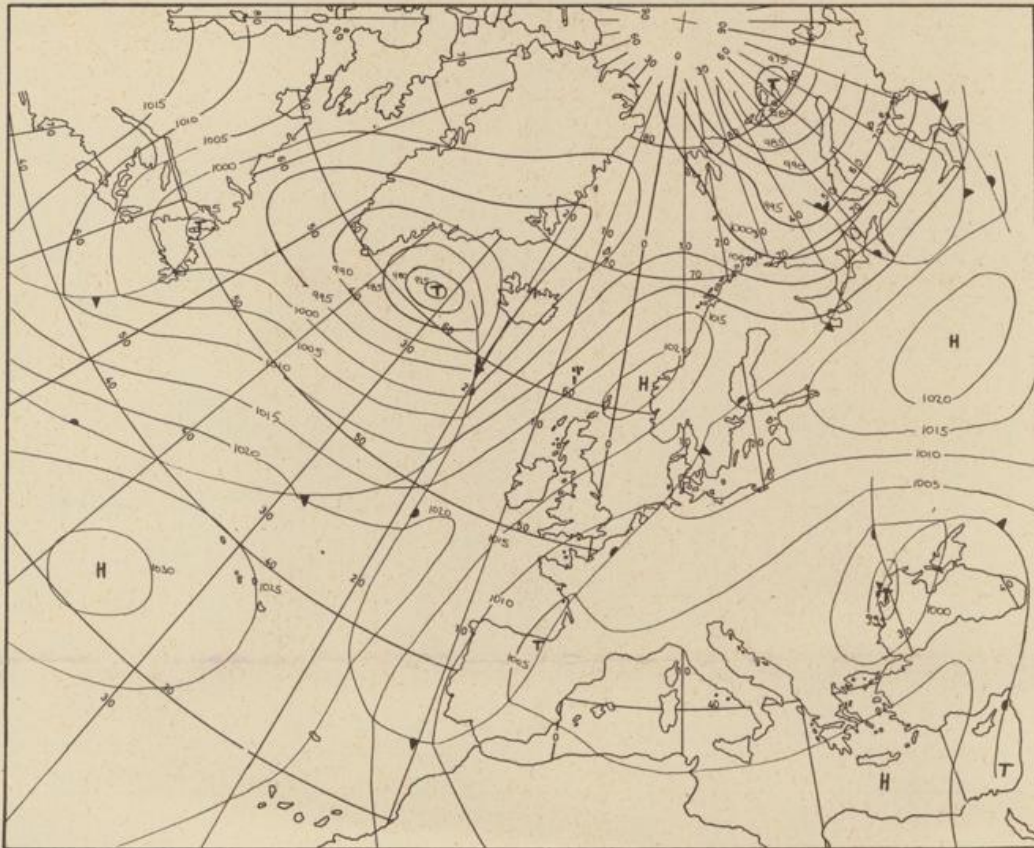
Bodenwetterkarte Vorhersage für den 13.4. 01 Uhr
