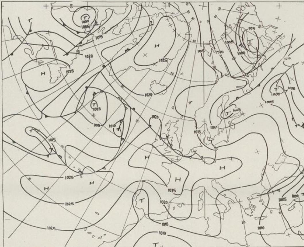
Bodenwetterkarte Vorhersage für den 25.07. 01 Uhr
