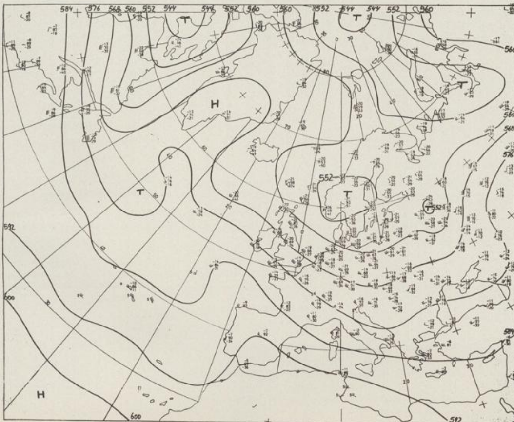
Höhenwetterkarte (Absolute Topographie 500 mb entsprechend ca. 5500 m Höhe) vom 24.07. 01 Uhr
