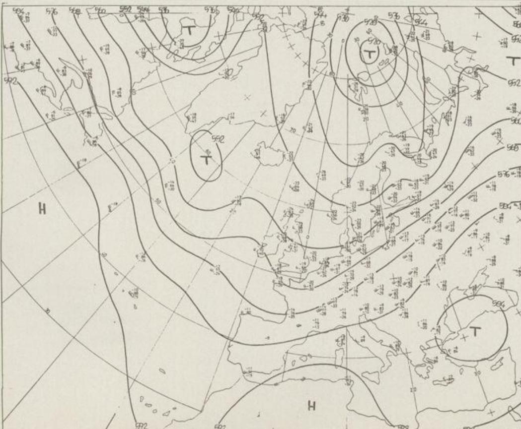
Höhenwetterkarte (Absolute Topographie 500 mb entsprechend ca. 5500 m Höhe) vom 04.08. 01 Uhr
