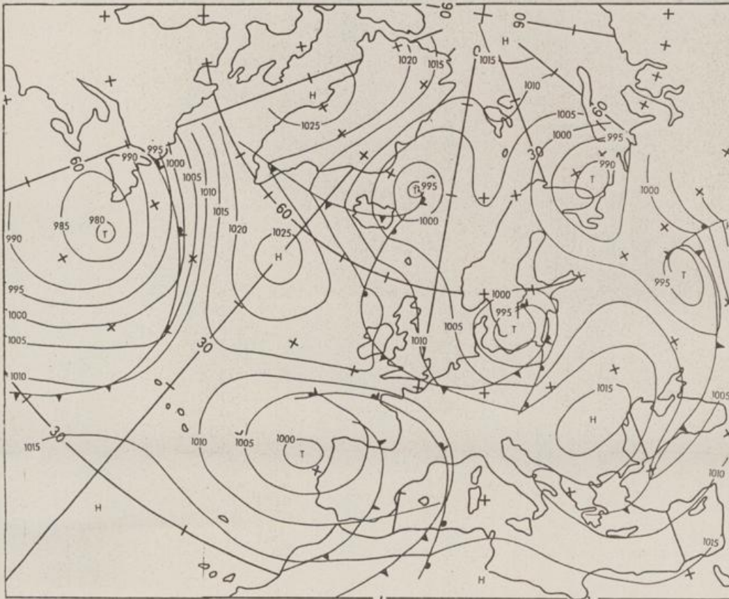
Bodenwetterkarte Vorhersage für den 12.11. 01 Uhr
