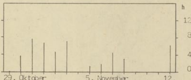
Sonnenscheindauer
