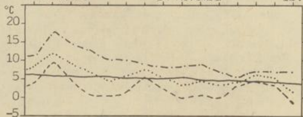
Lufttemperatur
