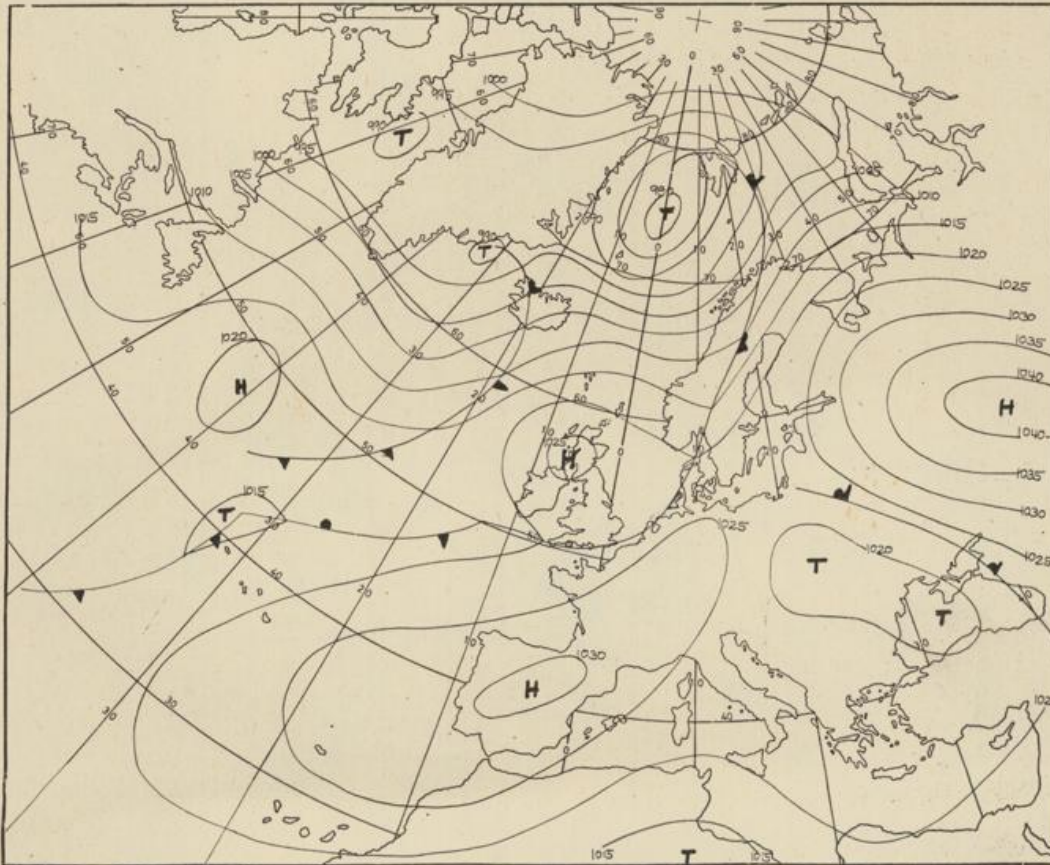
Bodenwetterkarte Vorhersage für den 17.11. 01 Uhr
