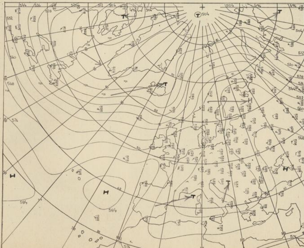
Höhenwetterkarte (Absolute Topographie 500 mb entsprechend ca. 5500 m Höhe) vom 16.11. 01 Uhr
