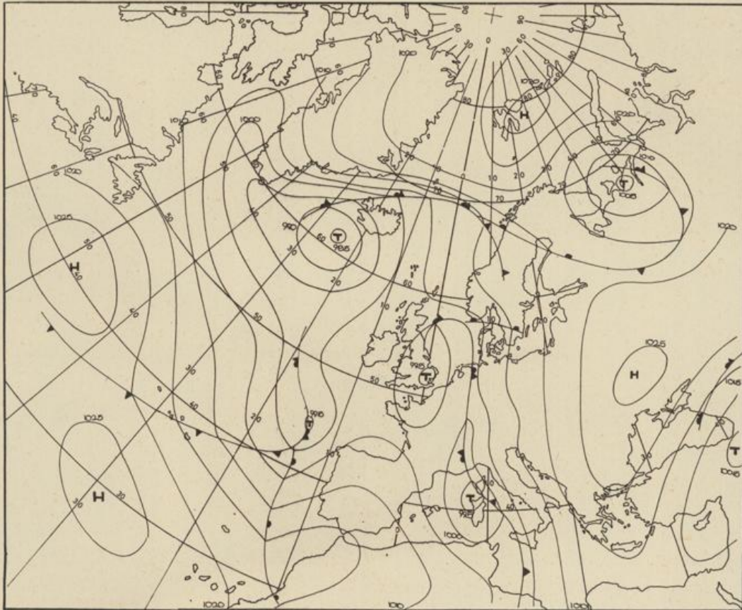
Bodenwetterkarte Vorhersage für den 26.10. 01 Uhr
