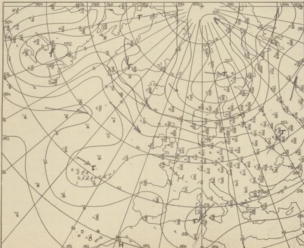
Höhenwetterkarte (Absolute Topographie 500 mb entsprechend ca. 5500 m Höhe) vom 8.9. 01 Uhr
