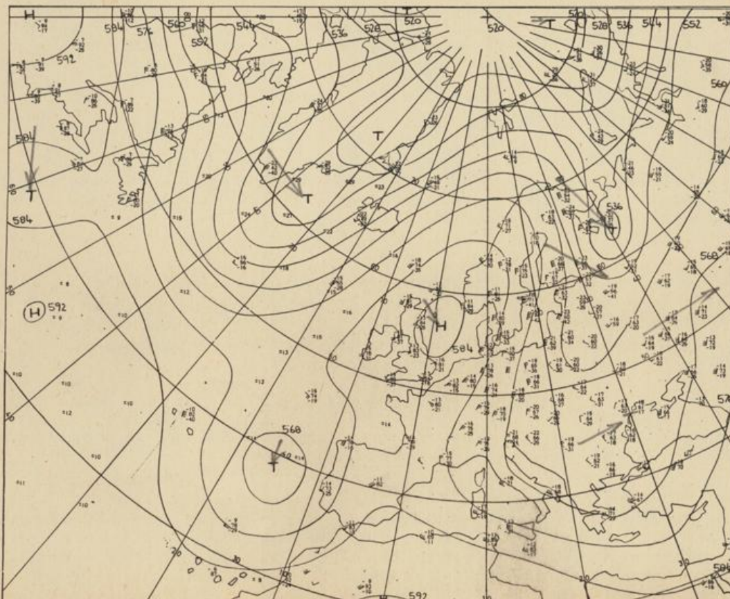
Höhenwetterkarte (Absolute Topographie 500 mb entsprechend ca. 5500 m Höhe) vom 21.8. 01 Uhr
