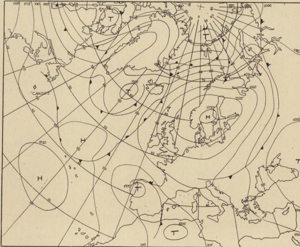
Bodenwetterkarte Vorhersage für den 22.8. 01 Uhr
