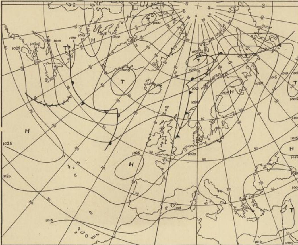
Bodenwetterkarte Vorhersage für den 13.8. 01 Uhr
