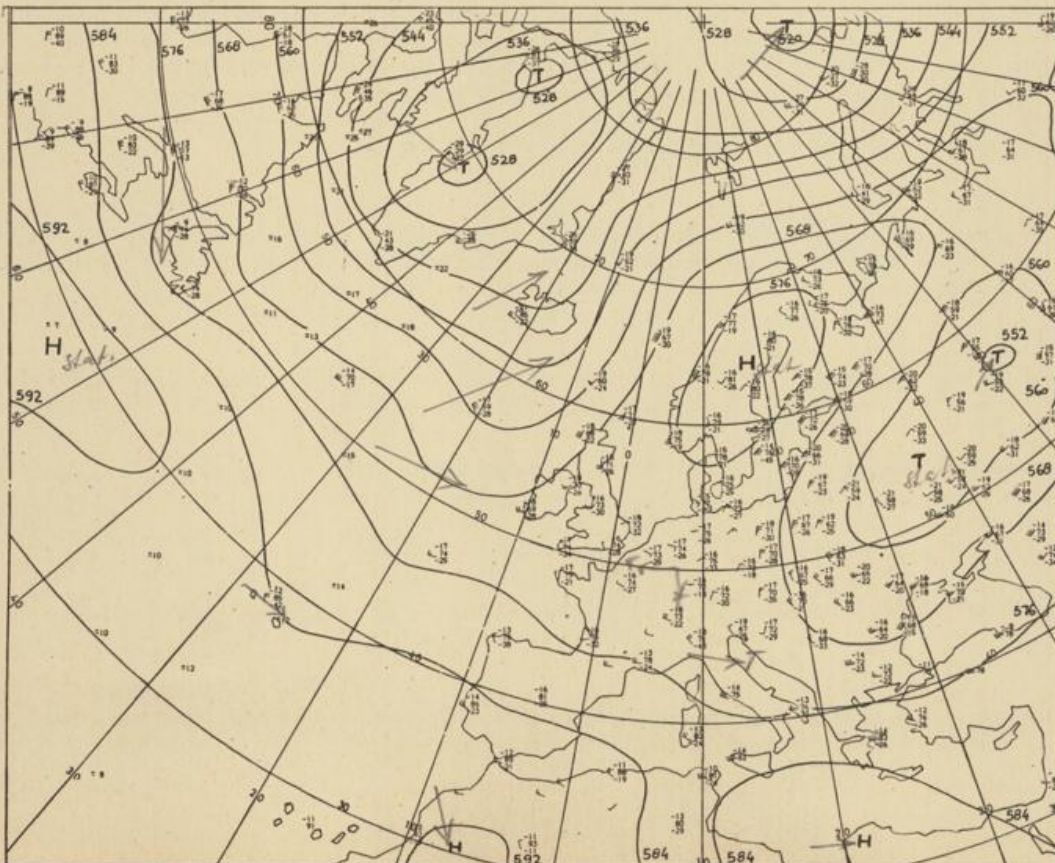
Höhenwetterkarte (Absolute Topographie 500 mb entsprechend ca. 5500 m Höhe) vom 12.8. 01 Uhr
