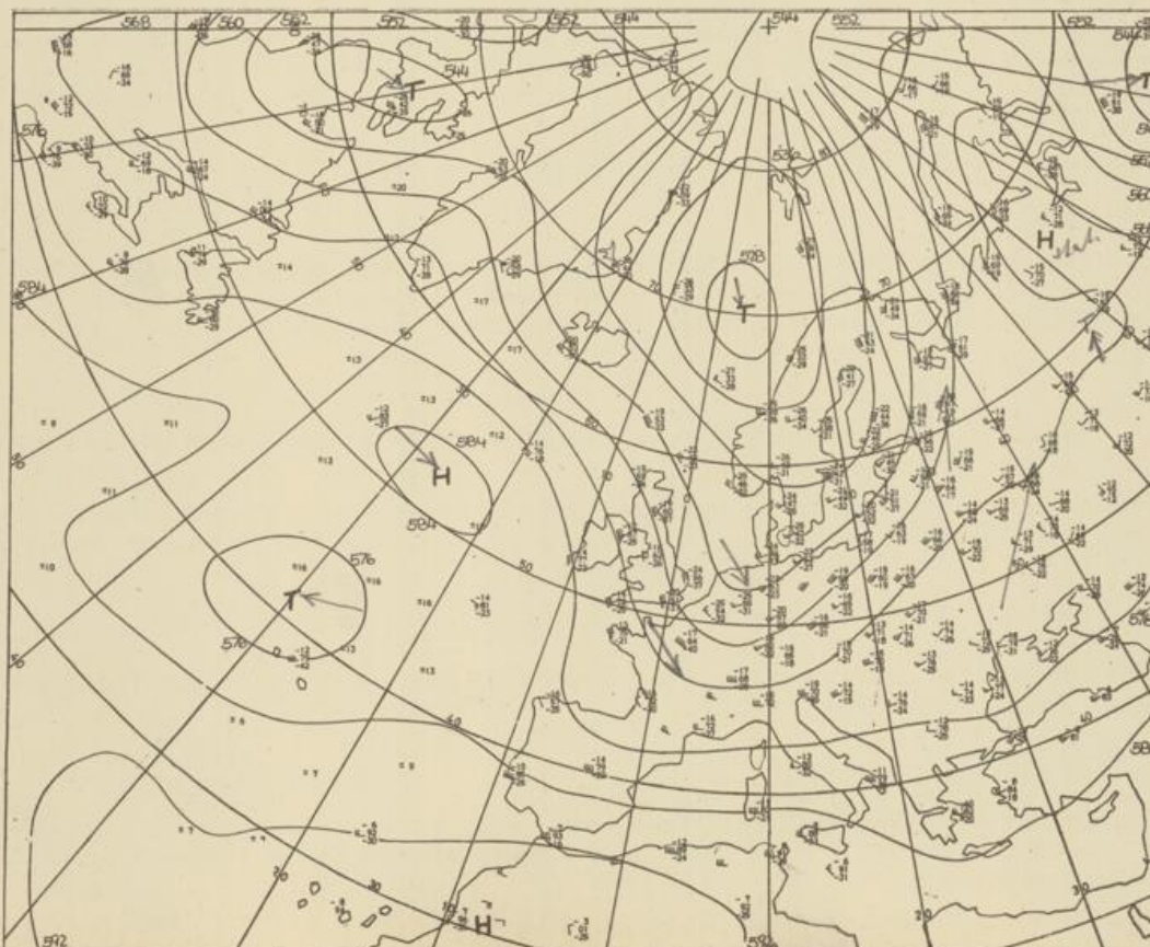
Höhenwetterkarte (Absolute Topographie 500 mb entsprechend ca. 5500 m Höhe) vom 1.8. 01 Uhr
