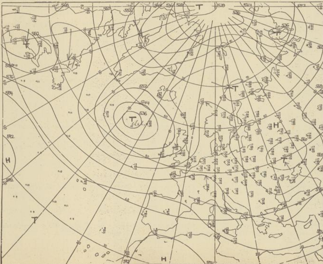
Höhenwetterkarte (Absolute Topographie 500 mb entsprechend ca. 5500 m Höhe) vom 14.7. 01 Uhr
