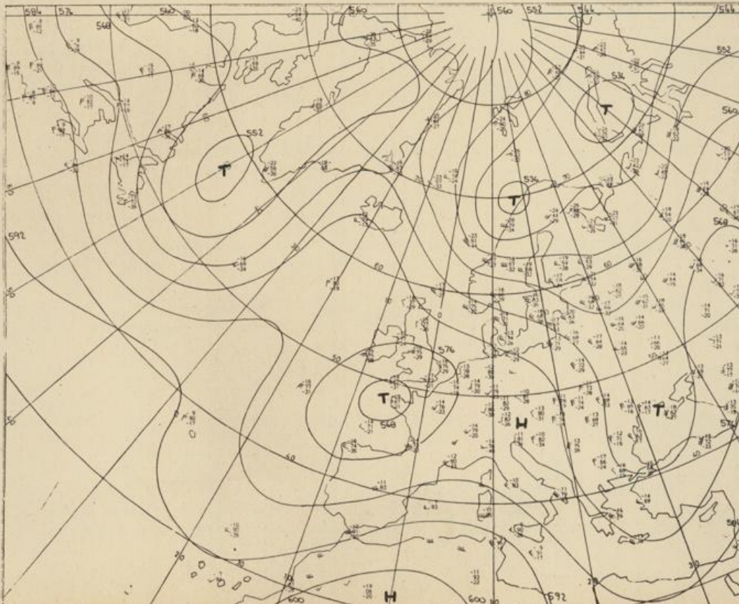
Höhenwetterkarte (Absolute Topographie 500 mb entsprechend ca. 5500 m Höhe) vom 13.7. 01 Uhr
