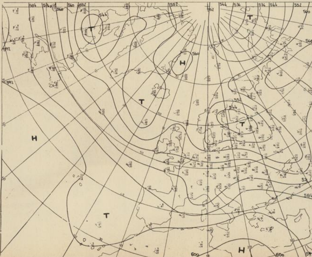
Höhenwetterkarte (Absolute Topographie 500 mb entsprechend ca. 5500 m Höhe) vom 17.7. 01 Uhr
