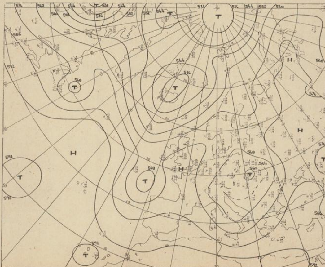
Höhenwetterkarte (Absolute Topographie 500 mb entsprechend ca. 5500 m Höhe) vom 2.8. 01 Uhr
