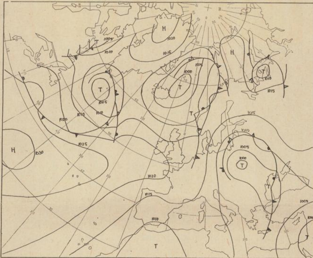
Bodenwetterkarte Vorhersage für den 3.8. 01 Uhr
