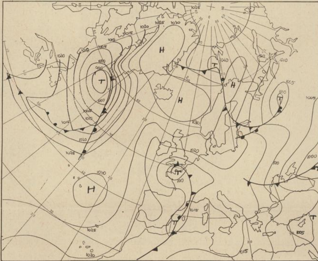
Bodenwetterkarte Vorhersage für den 17.8. 01 Uhr
