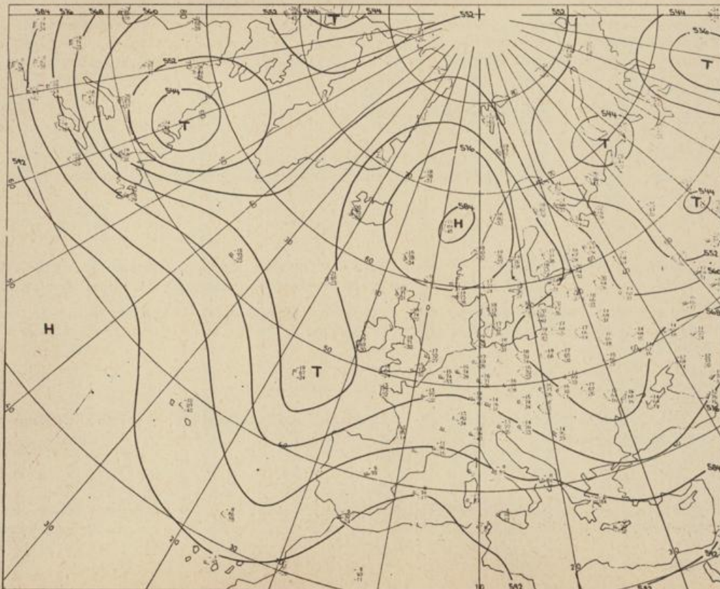
Höhenwetterkarte (Absolute Topographie 500 mb entsprechend ca. 5500 m Höhe) vom 16.8. 01 Uhr
