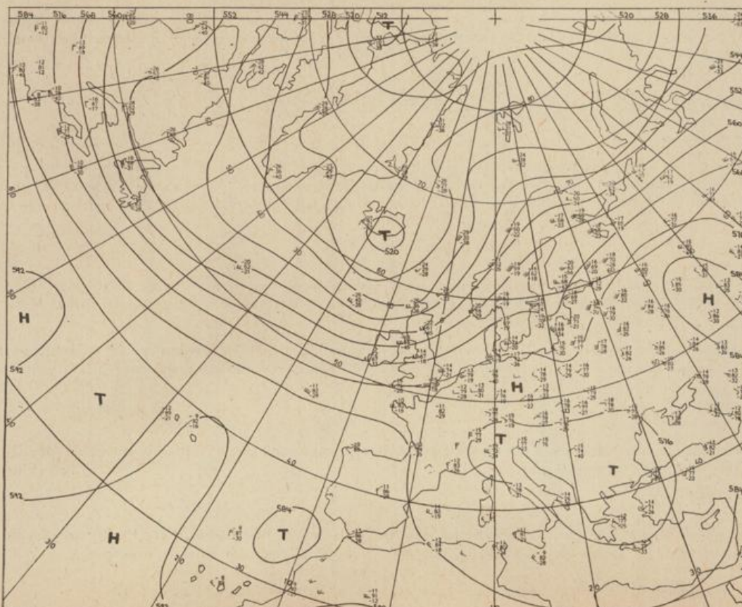
Höhenwetterkarte (Absolute Topographie 500 mb entsprechend ca. 5500 m Höhe) vom 5.9. 01 Uhr
