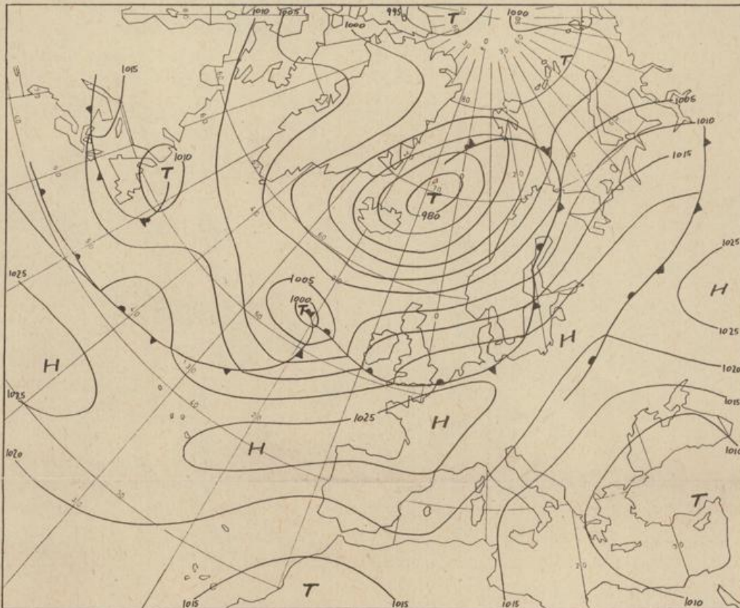
Bodenwetterkarte Vorhersage für den 6.9. 01 Uhr
