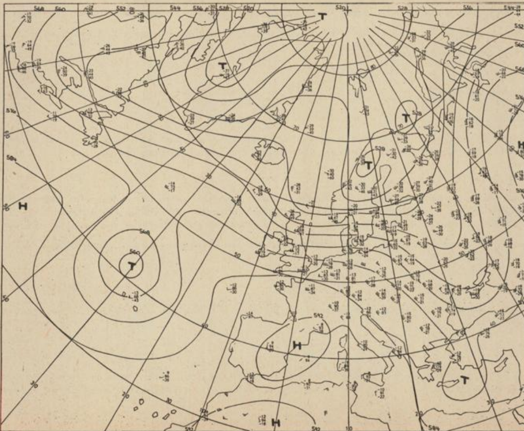
Höhenwetterkarte (Absolute Topographie 500 mb entsprechend ca. 5500 m Höhe) vom 12.9. 01 Uhr
