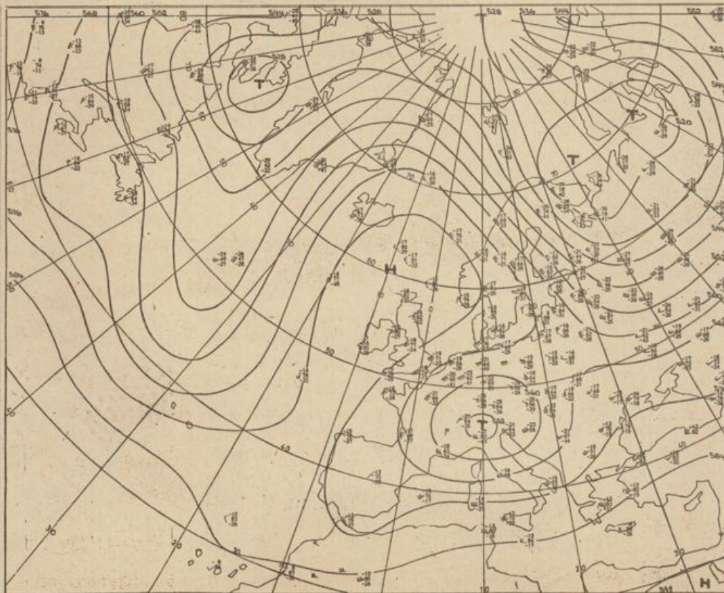
Höhenwetterkarte (Absolute Topographie 500 mb entsprechend ca. 5500 m Höhe) vom 19.9. 01 Uhr
