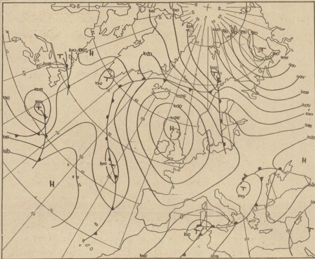
Bodenwetterkarte Vorhersage für den 20.9. 01 Uhr
