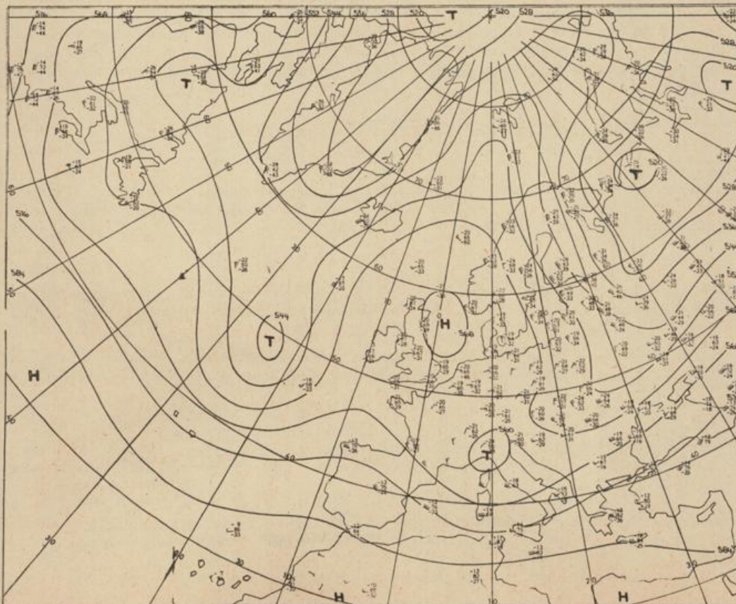
Höhenwetterkarte (Absolute Topographie 500 m entsprechend ca. 5500 m Höhe) vom 23.9. 01 Uhr
