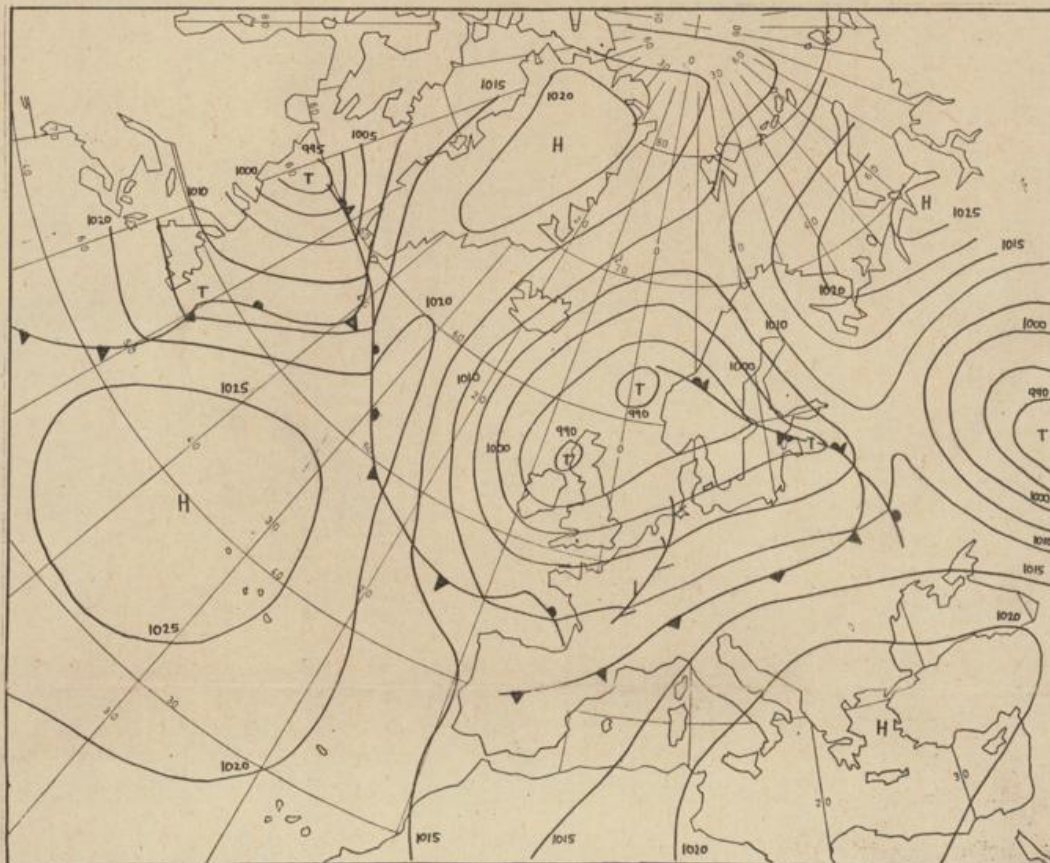
Bodenwetterkarte Vorhersage für den 6.10. 01 Uhr
