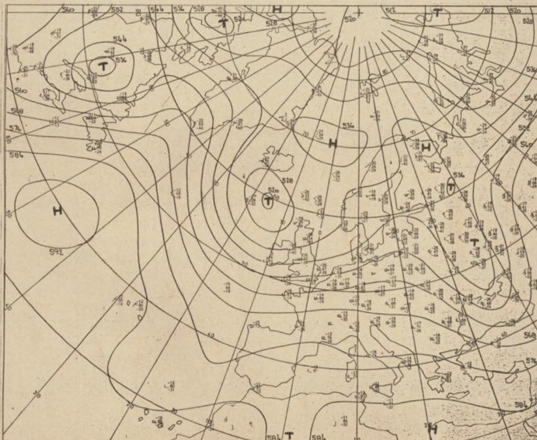
Höhenwetterkarte (Absolute Topographie 500 mb entsprechend ca. 5500 m Höhe) vom 5.10. 01 Uhr
