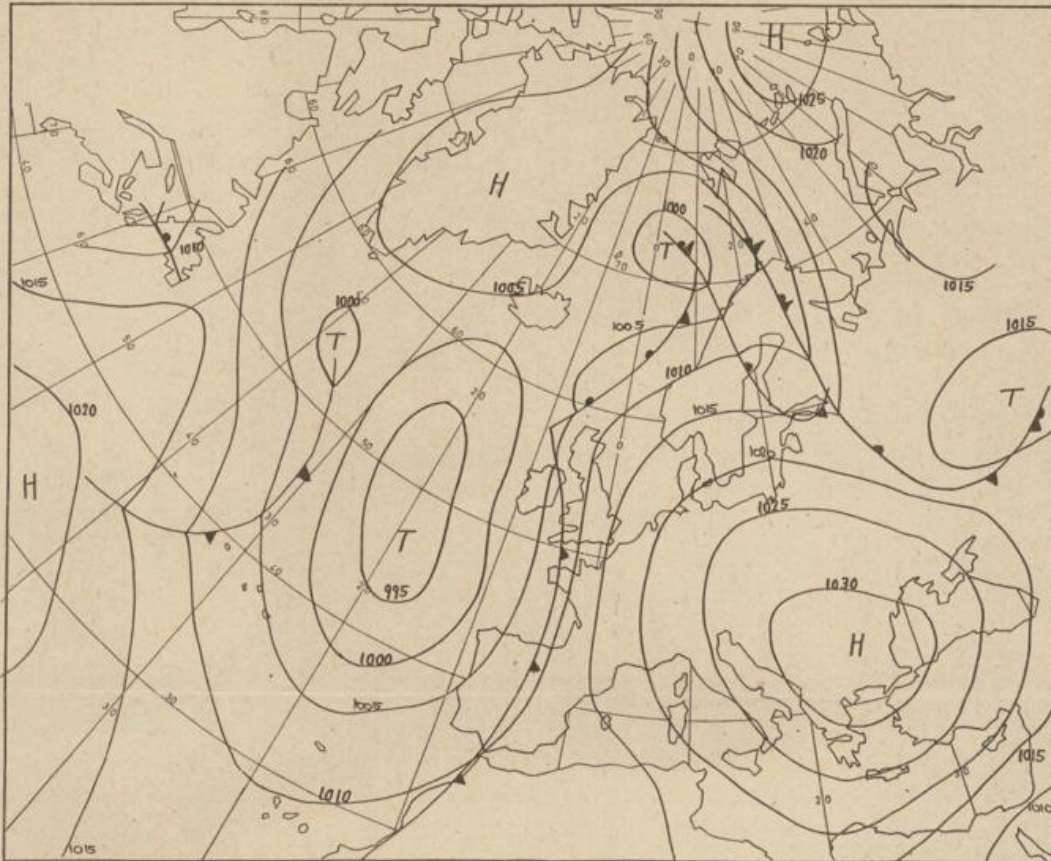
Bodenwetterkarte Vorhersage für den 18.10. 01 Uhr
