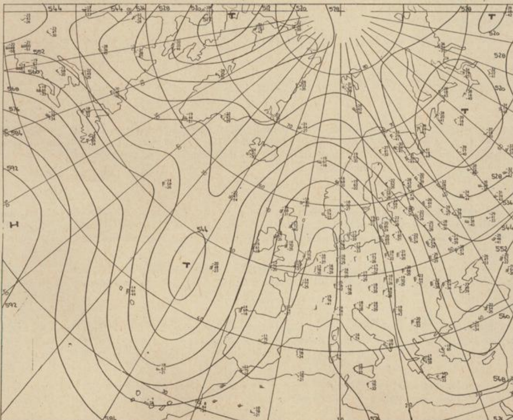
Höhenwetterkarte (Absolute Topographie 500 mb entsprechend ca. 5500 m Höhe) vom 17.10. 01 Uhr
