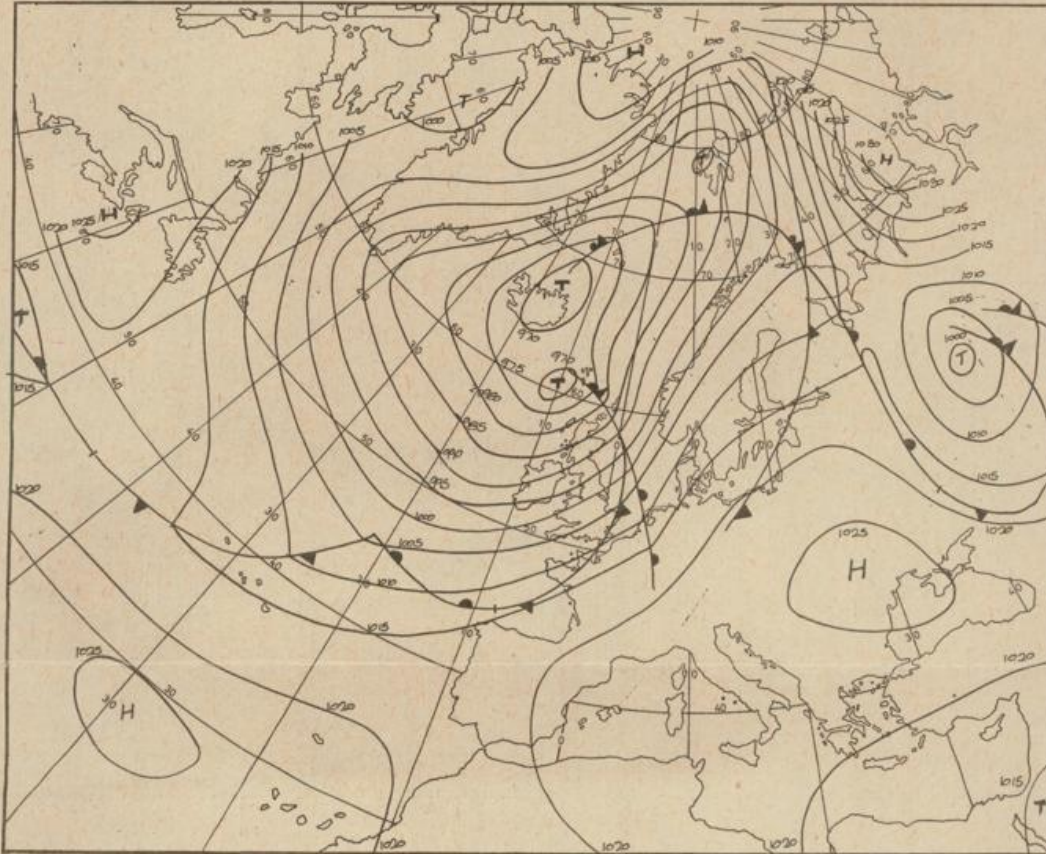
Bodenwetterkarte Vorhersage für den 31.10. 01 Uhr
