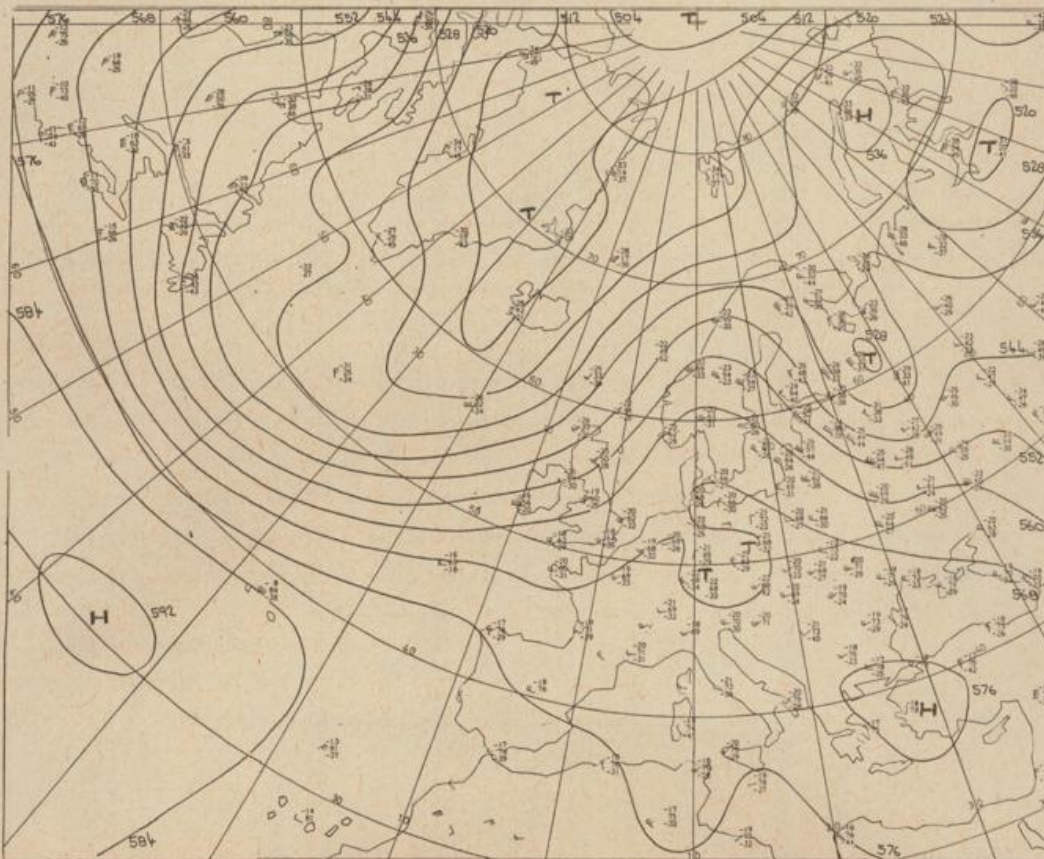
Höhenwetterkarte (Absolute Topographie 500 mb entsprechend ca. 5500 m Höhe) vom 30.10. 01 Uhr
