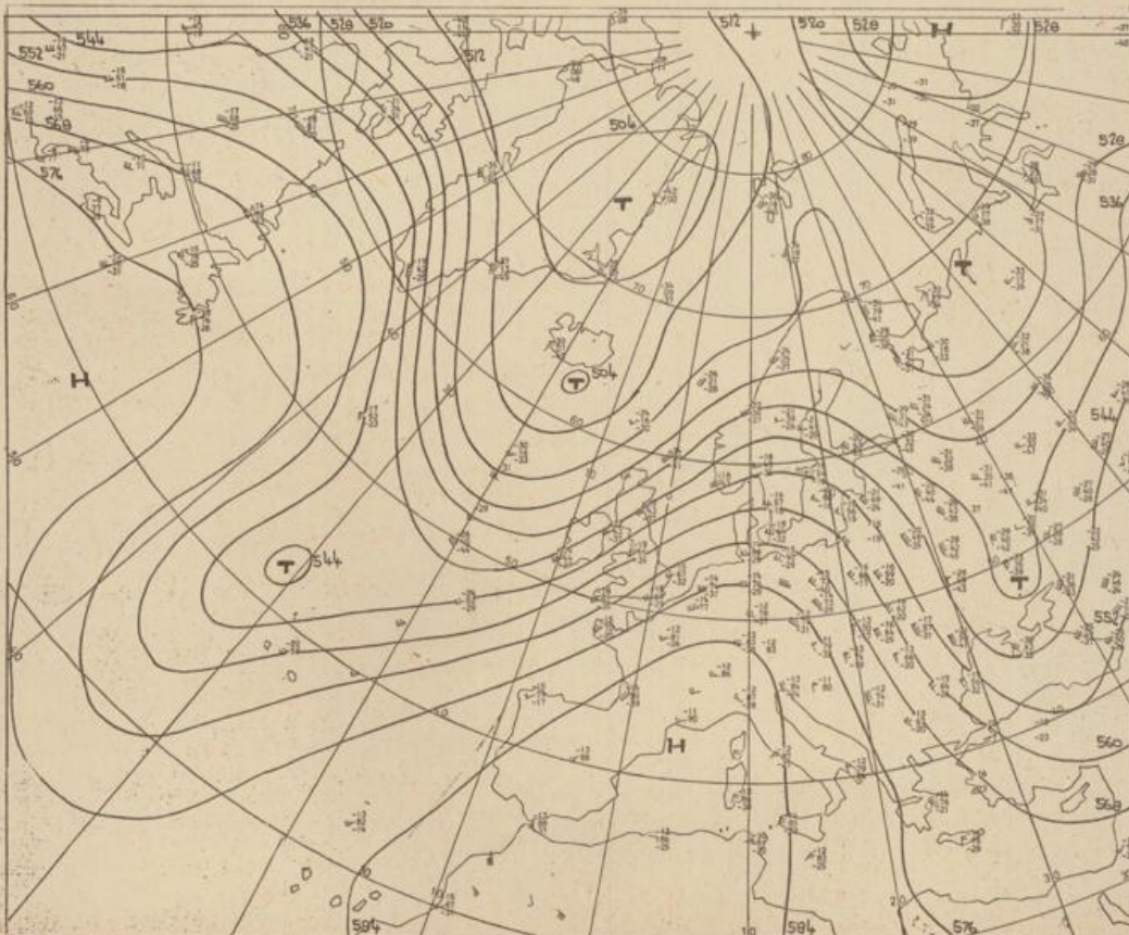
Höhenwetterkarte (Absolute Topographie 500 mb entsprechend ca. 5500 m Höhe) vom 11.11. 01 Uhr
