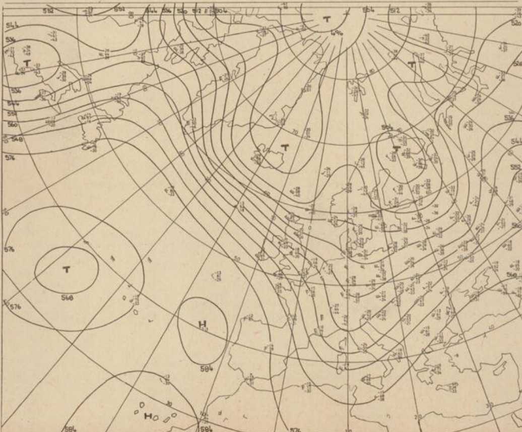
Höhenwetterkarte (Absolute Topographie 500 mb entsprechend ca. 5500 m Höhe) vom 14.11. 01 Uhr
